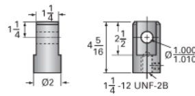
Clevis End (optional): 9001-00-03
