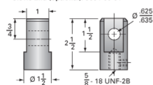
Clevis End (optional): 9001-00-01
