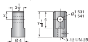
Clevis End (optional): 9001-00-16
