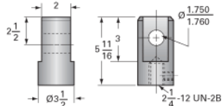
Clevis End (optional): 9001-00-07
