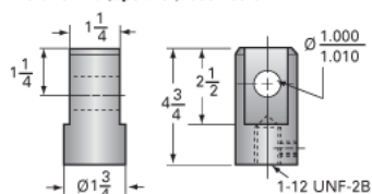
Clevis End (optional): 9001-00-02
