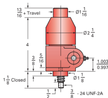
Clevis End (optional): 9001-00-12
