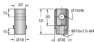
Clevis End (optional): 9001-EM-12
