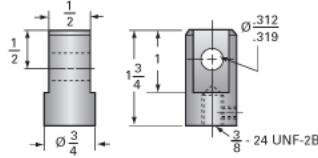
Clevis End (optional): 9001-00-12
