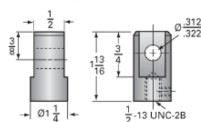
Clevis End (optional): 9001-00-11
