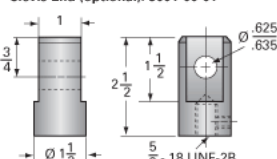
Clevis End (optional): 9001-00-01
