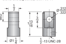
Clevis End (optional): 9001-00-11
