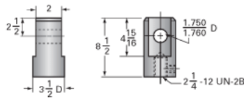
Clevis End (optional): 9001-00-08
