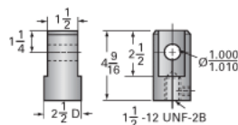
Clevis End (optional): 9001-00-09
