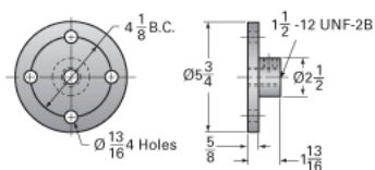
Top Plate (optional): 9000-00-01
