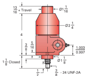
Clevis End (optional): 9001-00-12
